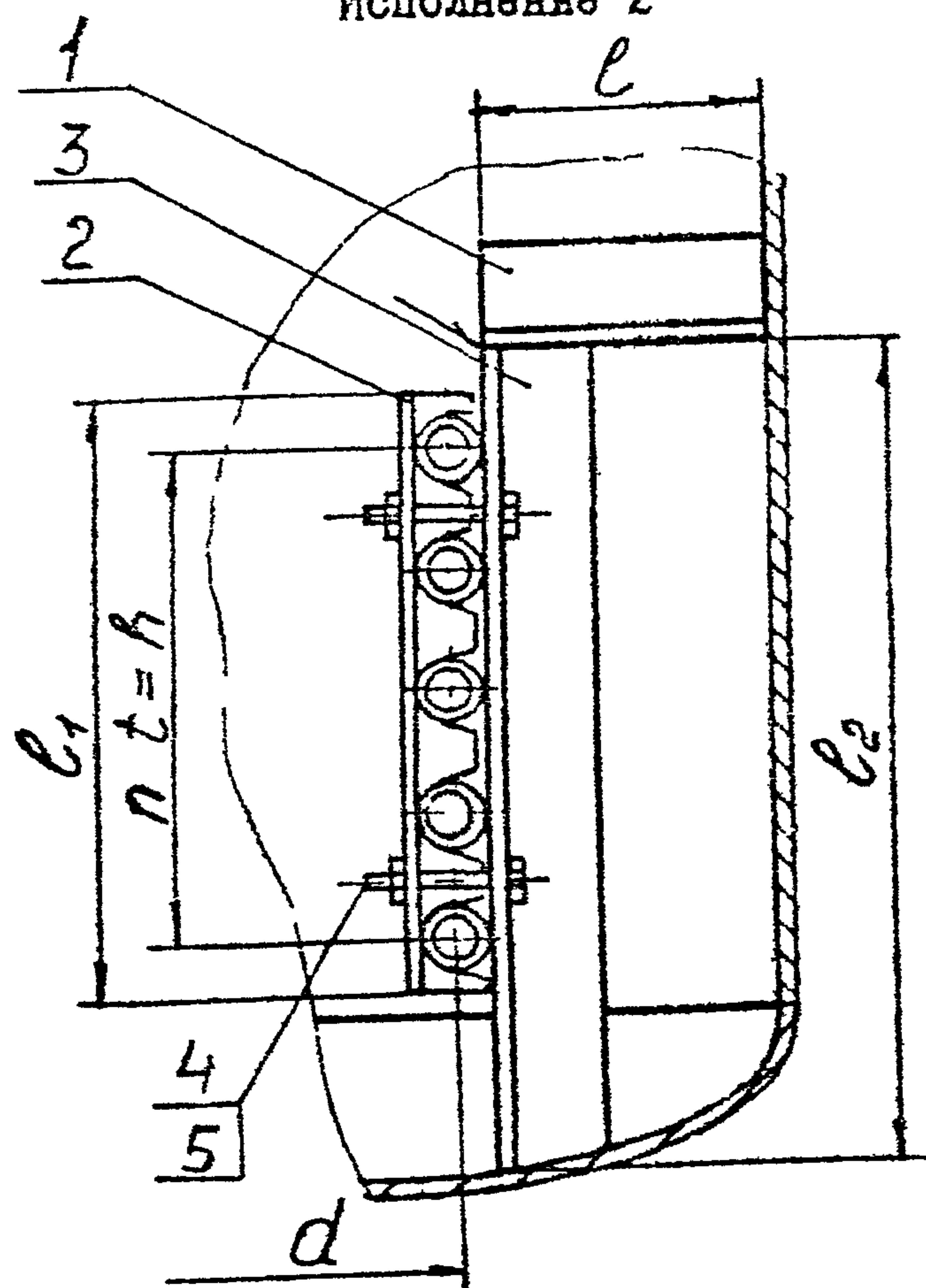
А-А Исполнение 2
