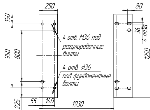
План расположения отверстий под фундаментные болты и регулировочные винты
