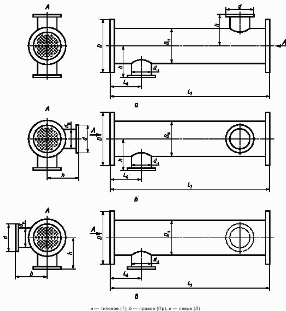
Рисунок 9 — Варианты исполнения блоков-секций по расположению патрубков
