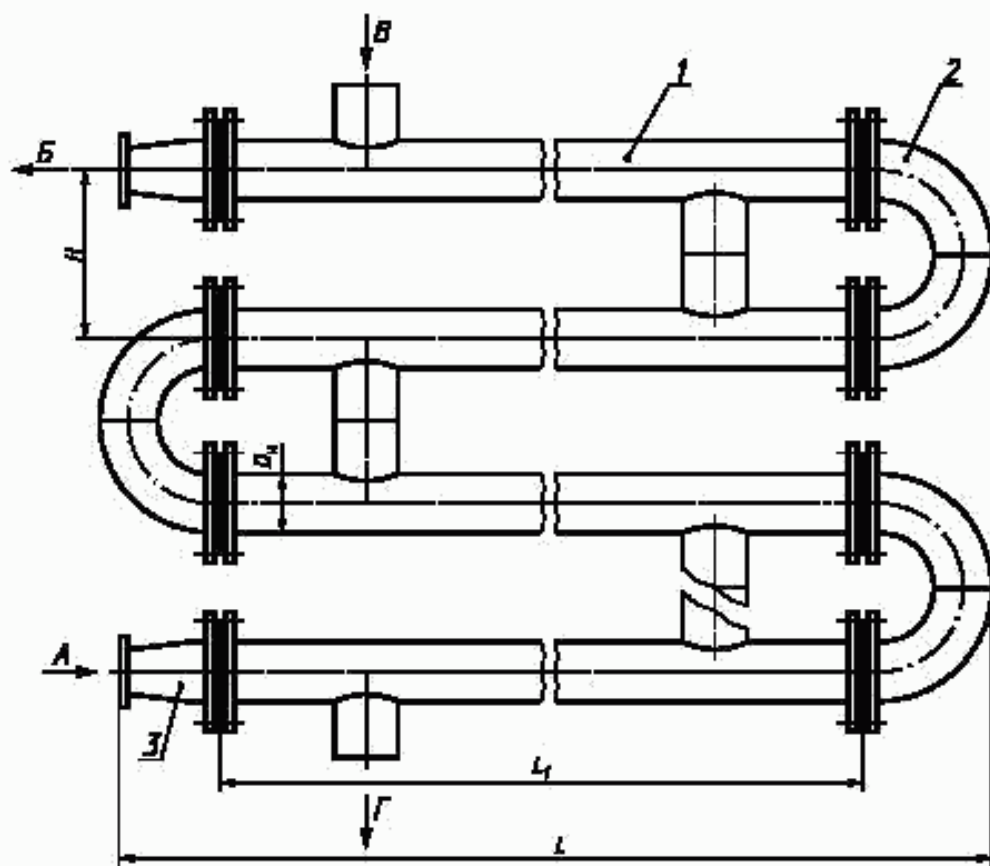
Рисунок 3 — Подогреватель из четырех блоков-секций типа ПВ2 с типовым расположением патрубков без компенсатора на корпусе
