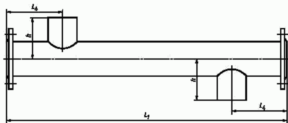
Рисунок 8 — Блок-секция типа PB2 без компенсатора и с типовым расположением патрубков
