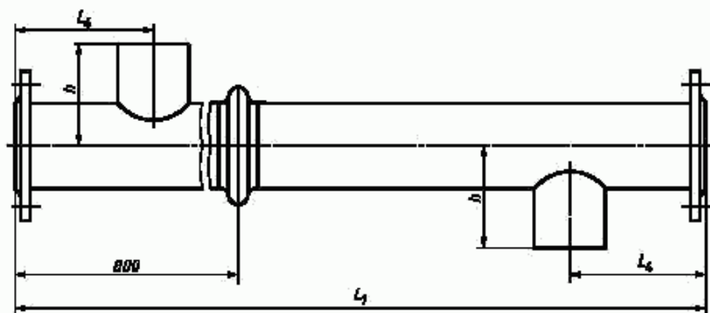
Рисунок 7 — Блок-секция PB2K с компенсатором и с типовым расположением патрубков
